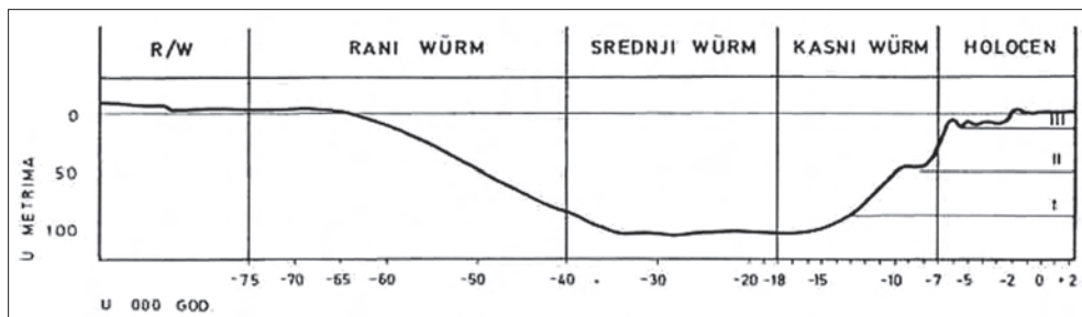
Slika 4. Gladina Sredozemskega morja med zadnjimi ledenimi dobami in otoplitvijo [4]
