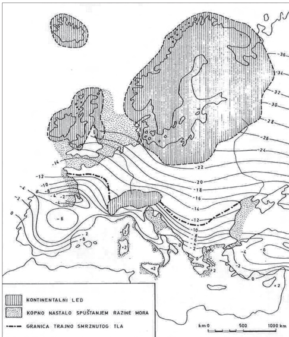
Slika 3. Srednje januarske temperature v maksimumu würma, s kontinentalnim ledom in povečanjem kopne površine zaradi znižanje Sredozemskega morja [4].
