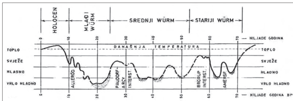
Slika 2. Prikaz srednje letne temperature v Srednji Evropi v würmu in holocenu [4]
